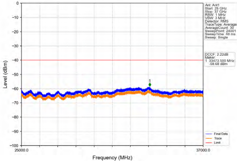
Band48_20MHz_QPSK_HCH_3690MHz_RB_1_99_NTNV
