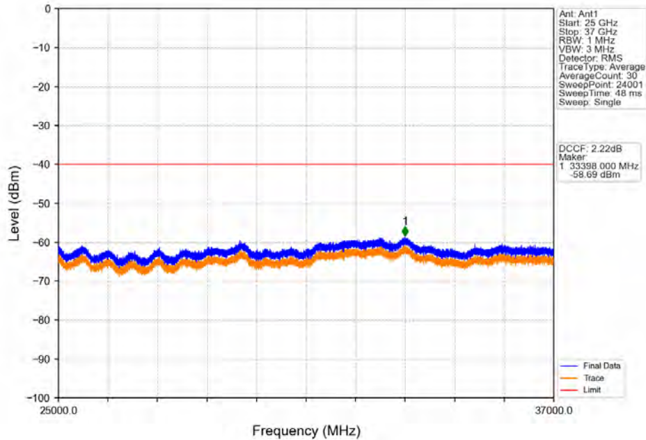
Band48_15MHz_QPSK_HCH_3692.5MHz_RB_1_74_NTNV
