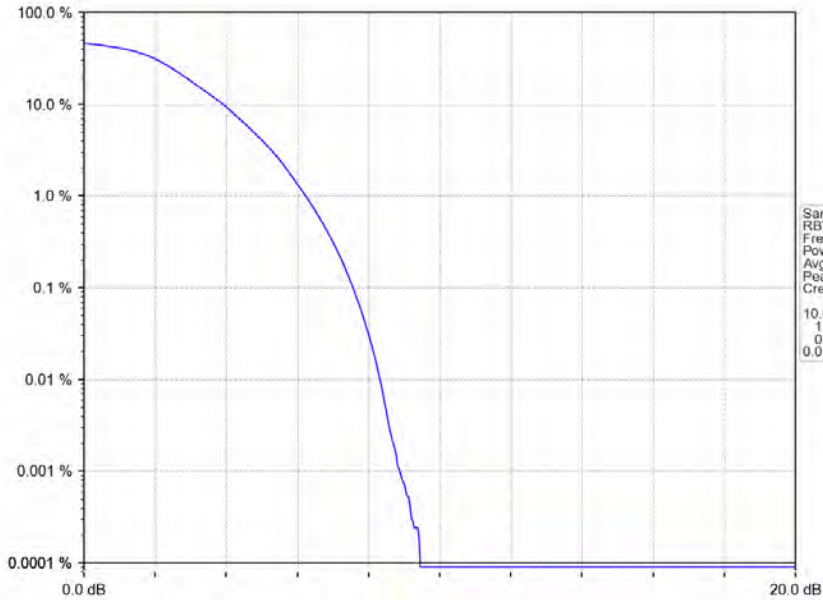
Band48_20MHz_QPSK_HCH_3690MHz_RB_100_0_NTNV
