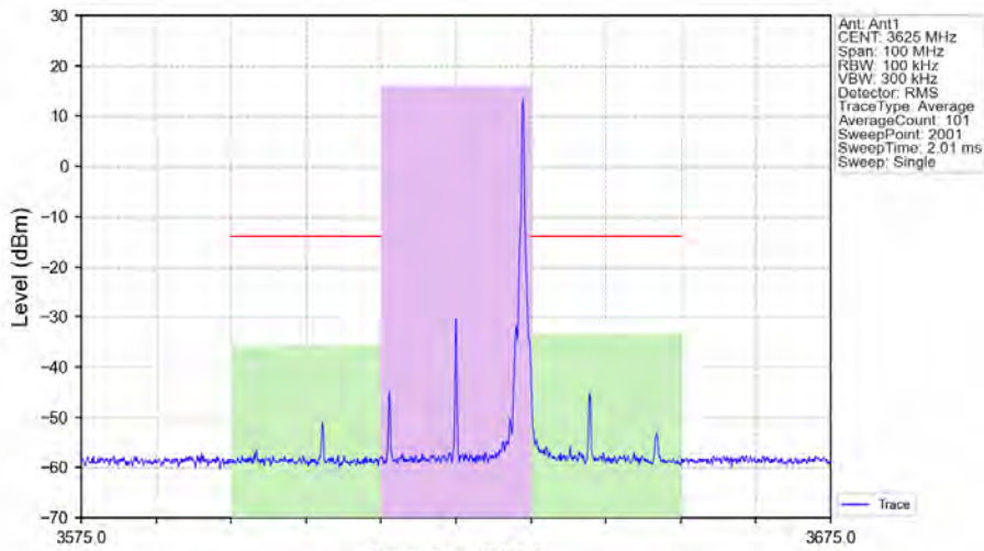
Band48_20MHz_QPSK_MCH_3625MHz_RB_1_99_NTNV
