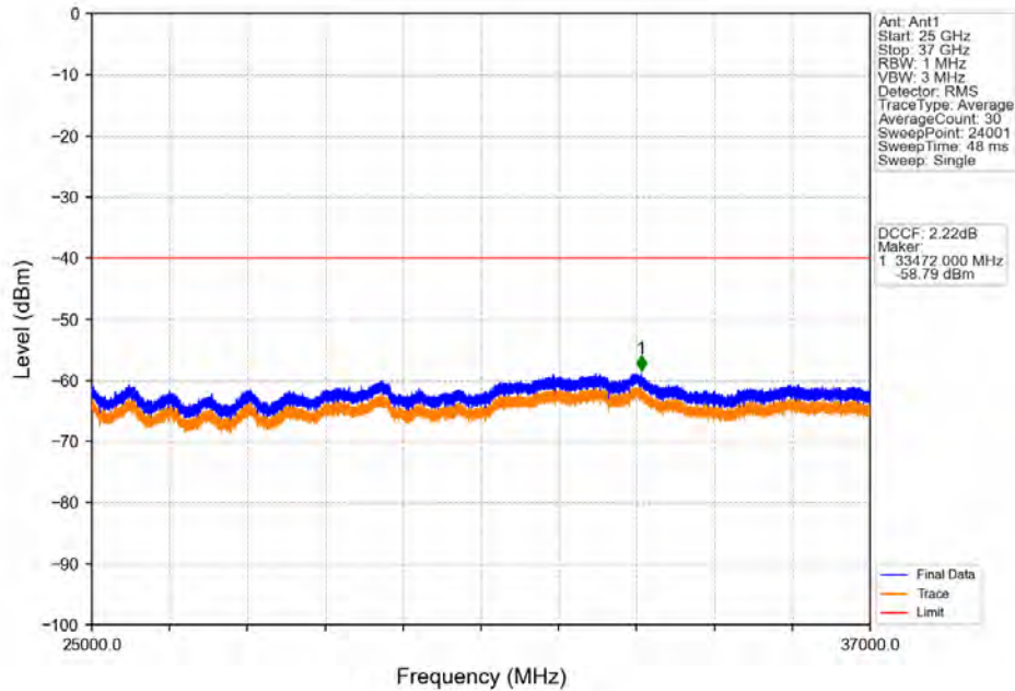
Band48_10MHz_QPSK_HCH_3695MHz_RB_1_49_NTNV
