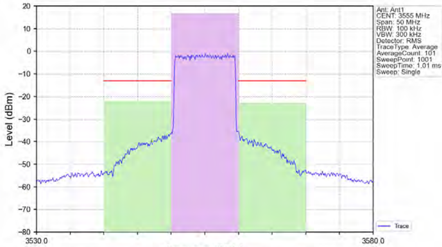
Band48_10MHz_QPSK_LCH_3555MHz_RB_50_0_NTNV
