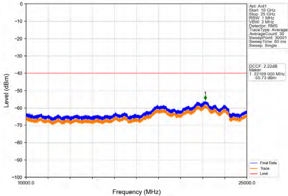
Band48_10MHz_QPSK_LCH_3555MHz_RB_1_0_NTNV
