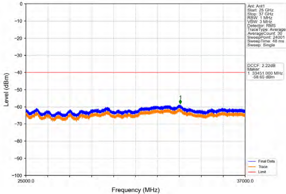
Band48_5MHz_QPSK_HCH_3697.5MHz_RB_1_24_NTNV
