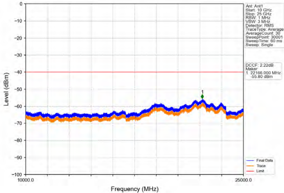
Band48_20MHz_QPSK_MCH_3625MHz_RB_1_0_NTNV
