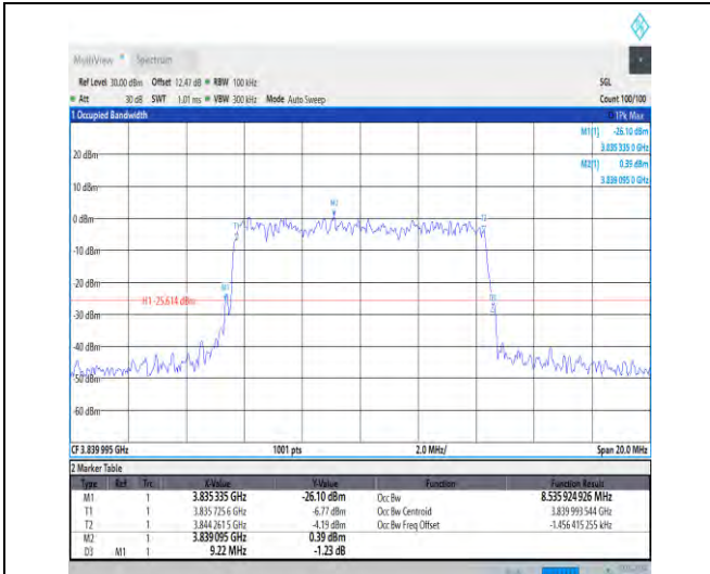
1-N77-3700-3980-30-10-M-9-CP-256QAM-Outer_Fu ll-24@0-Ant3-8.536-9.220-≤10-PASS
