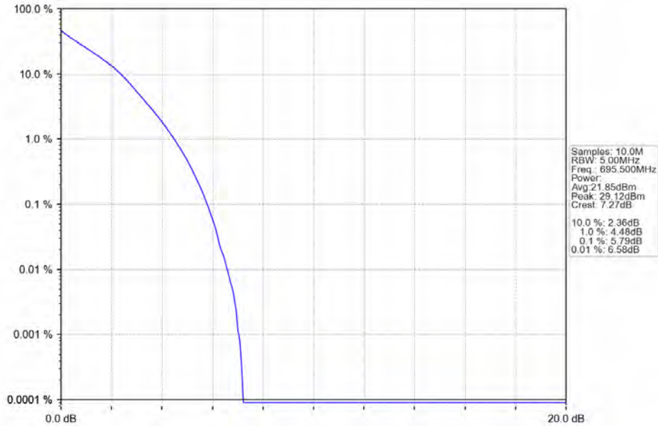
Band71_5MHz_QPSK_HCH_695.5MHz_RB_25_0_NTNV
