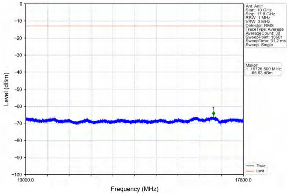
Band66_20MHz_QPSK_LCH_1720MHz_RB_100_0_NTNV
