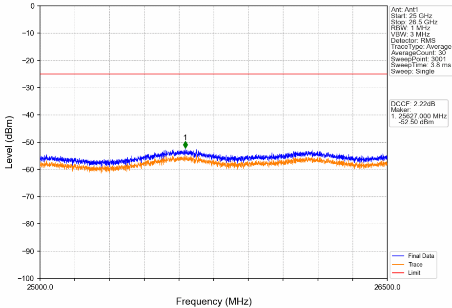
Band41_15MHz_QPSK_HCH_2682.5MHz_RB_1_74_NTNV
