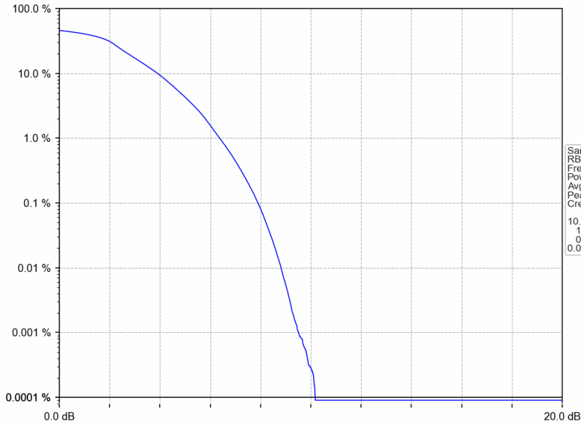
Band41 20MHz_QPSK_HCH_2680MHz_RB_100_0_NTNV
