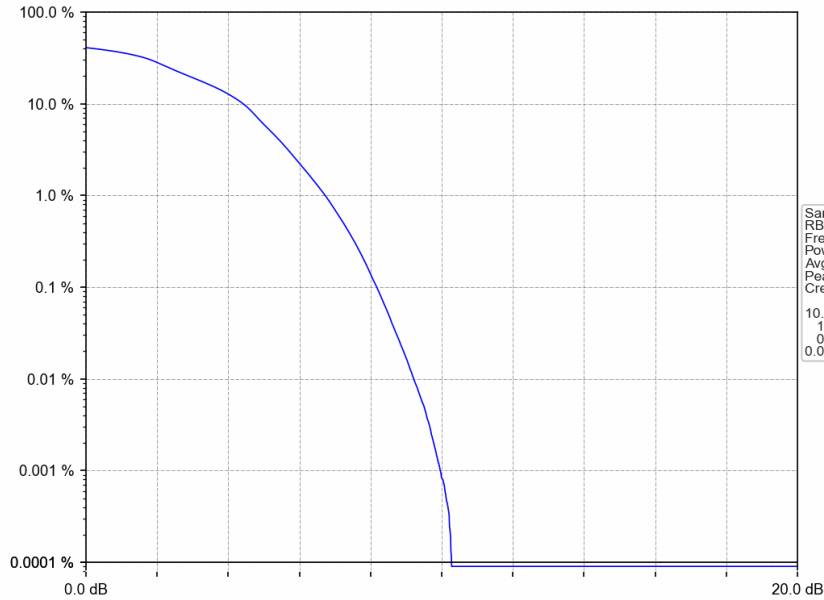
Band41_20MHz_16QAM MCH_2593MHz_RB_100_0_NTNV
