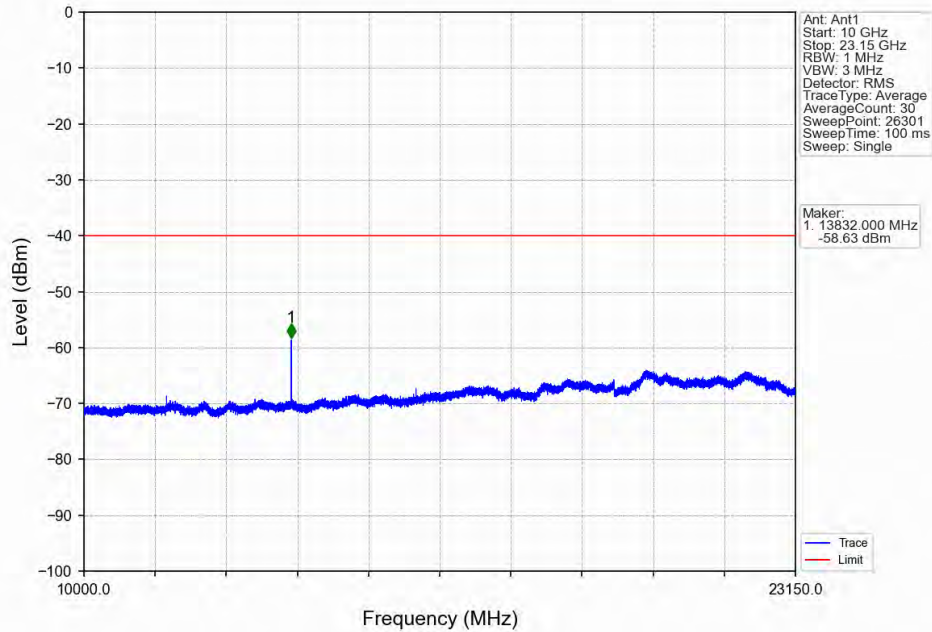
Band30_5MHz_QPSK_LCH_2307.5MHz_RB_25_0_NTNV
