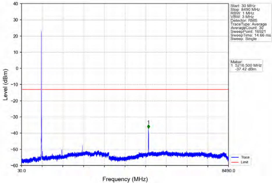
Band26b_10MHz_QPSK_HCH_844MHz_RB_1_49_NTNV
