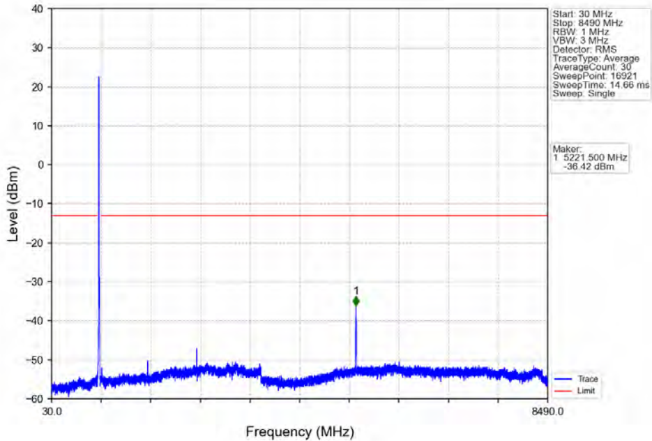
Band26b_15MHz_QPSK_HCH_841.5MHz_RB_1_74_NTNV
