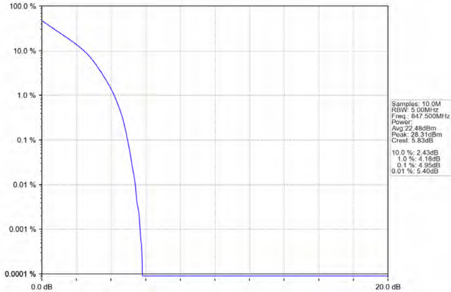
Band26b_3MHz_QPSK_HCH_847.5MHz_RB_15_0_NTNV
