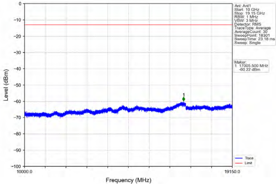
Band25_10MHz_QPSK_LCH_1855MHz_RB_50_0_NTNV
