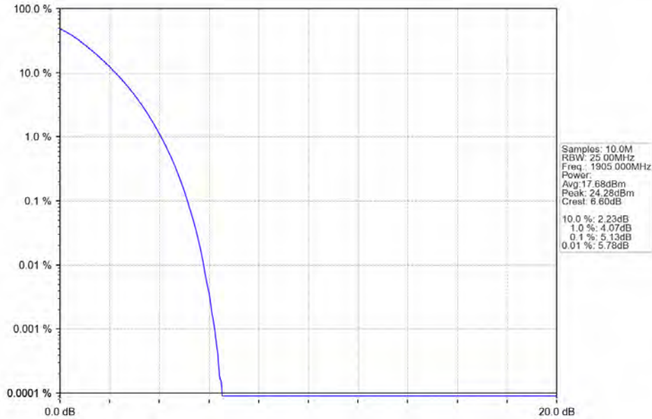
Band25_20MHz_QPSK_HCH_1905MHz_RB_100_0_NTNV
