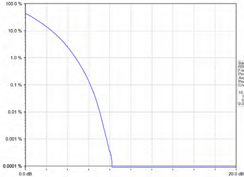
Band4_20MHz_QPSK_HCH_1745MHz_RB_100_0_NTNV
