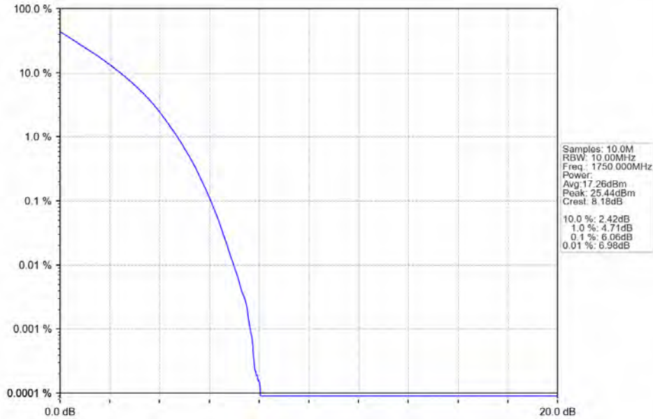
Band4 10MHz_QPSK_HCH_1750MHz_RB_50_0_NTNV
