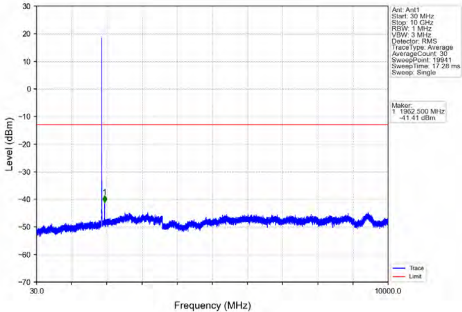
Band2_10MHz_QPSK_MCH_1880MHz_RB_1_0_NTNV
