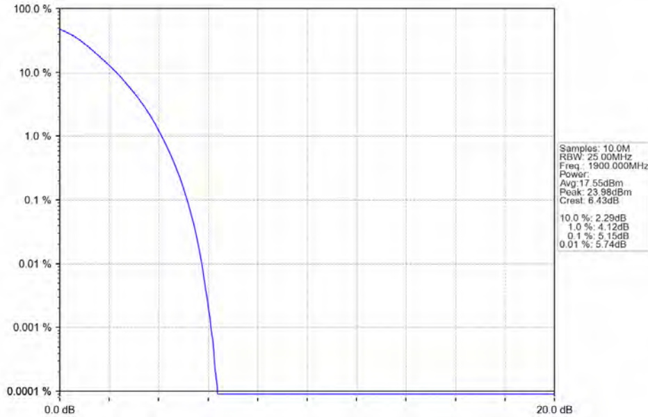
Band2_20MHz_QPSK_HCH_1900MHz_RB_100_0_NTNV
