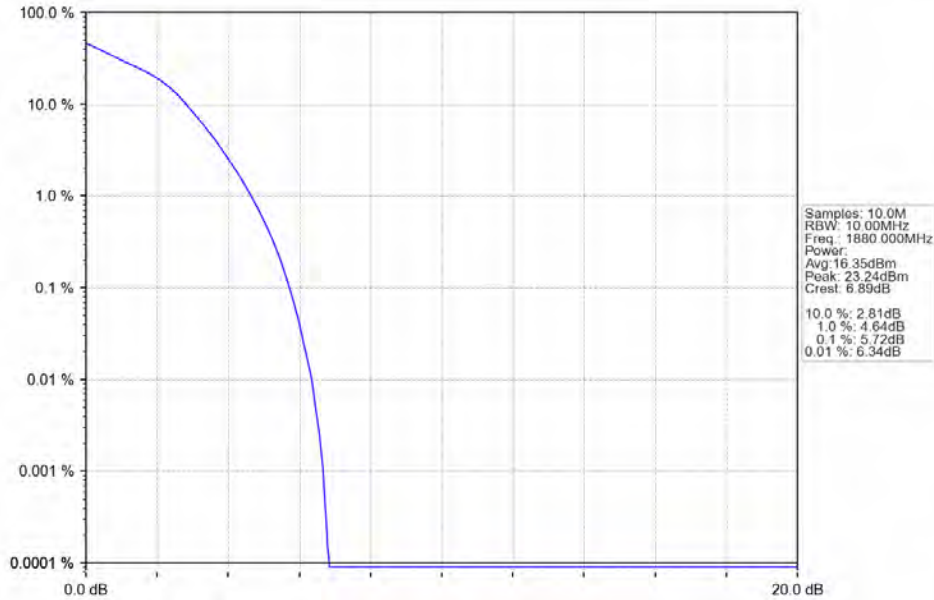
Band2_10MHz_16QAM_MCH_1880MHz_RB_50_0_NTNV
