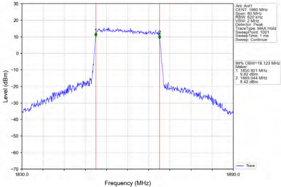
Band2_20MHz_16QAM_LCH_1860MHz_RB_100_0_NTNV
