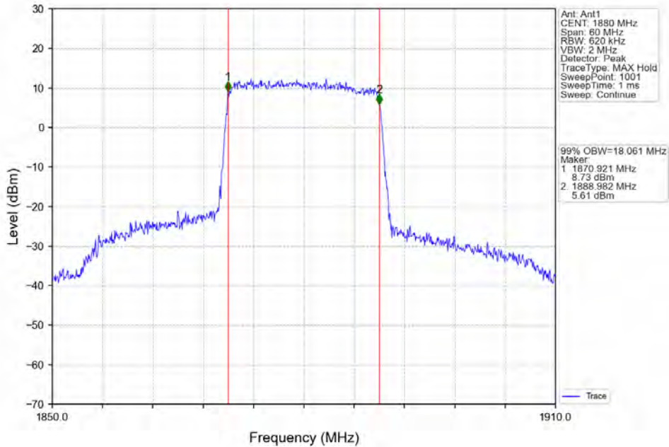
Band2_20MHz_64QAM_MCH_1880MHz_RB_100_0_NTNV
