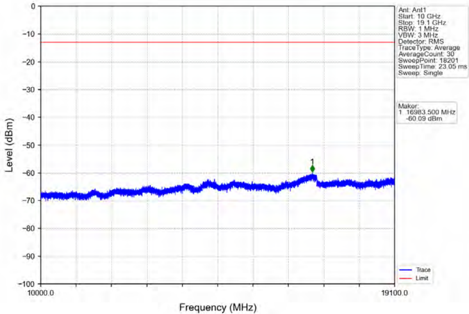
Band2_20MHz_QPSK_LCH_1860MHz_RB_100_0_NTNV
