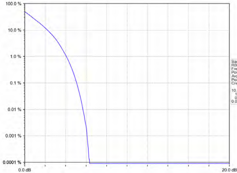
Band2_10MHz_QPSK_HCH_1905MHz_RB_50_0_NTNV
