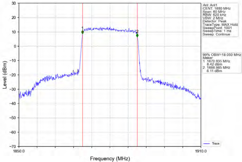
Band2_20MHz_16QAM_MCH_1880MHz_RB_100_0_NTNV
