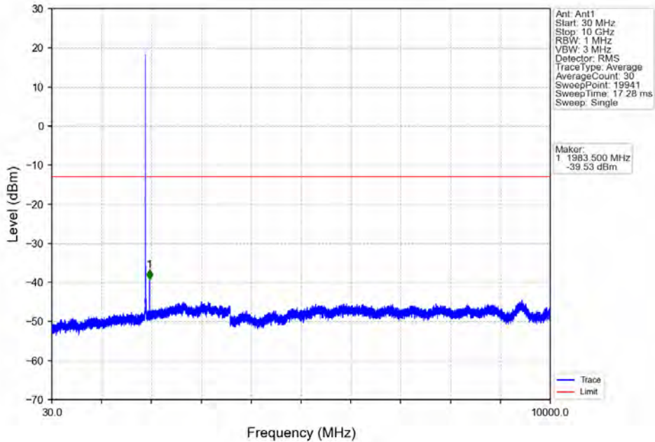
Band2_10MHz_QPSK_HCH_1905MHz_RB_1_0_NTNV
