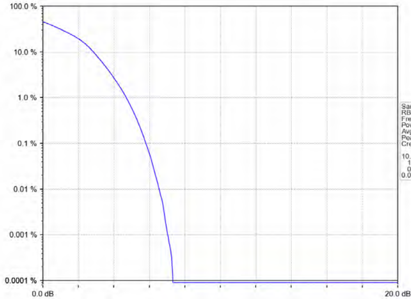
Band2_20MHz_16QAM_MCH_1880MHz_RB_100_0_NTNV
