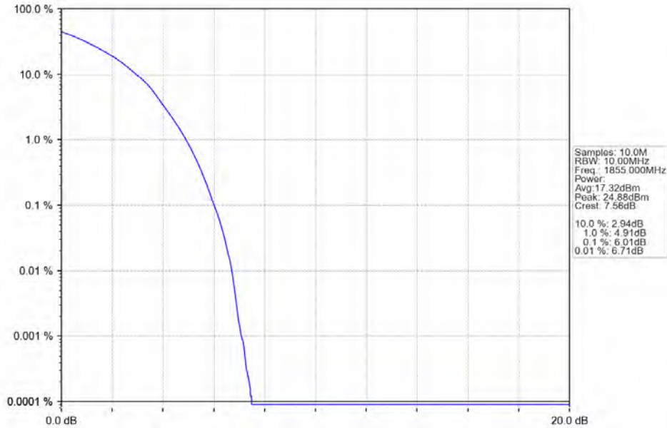
Band2_10MHz_64QAM_LCH_1855MHz_RB_50_0_NTNV
