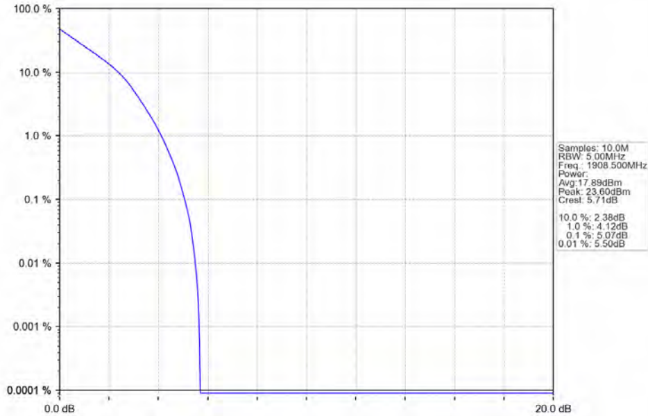
Band2_3MHz_QPSK_HCH_1908.5MHz_RB_15_0_NTNV
