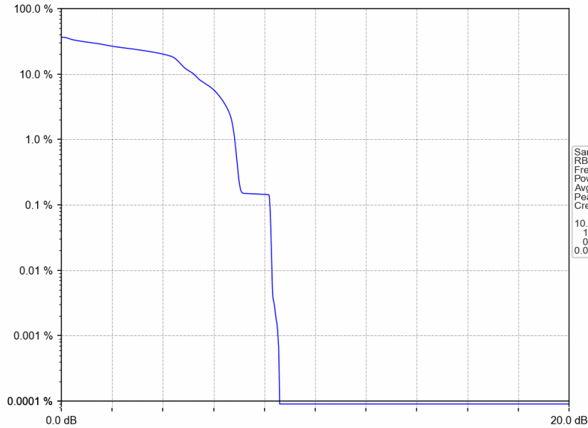
PCS1900_EGPRS_HCH_1909.8MHz_4 TX Slots_NTNV
