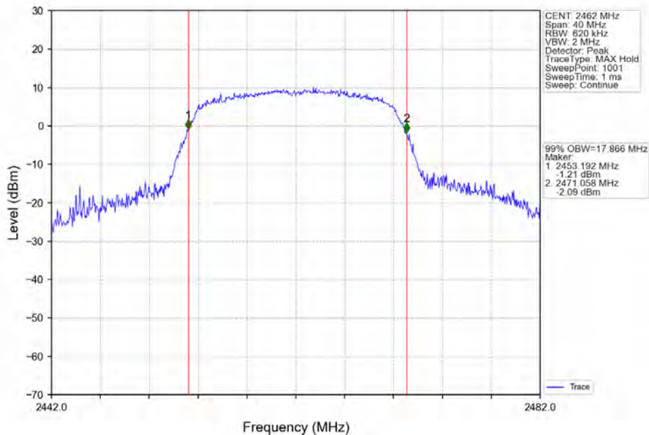
802.11g_HCH_2462MHz_Ant7 (SISO)_NTNV
