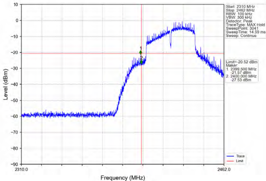
802.11n(HT40)_LCH_2422MHz_Ant7 (SISO)_NTNV
