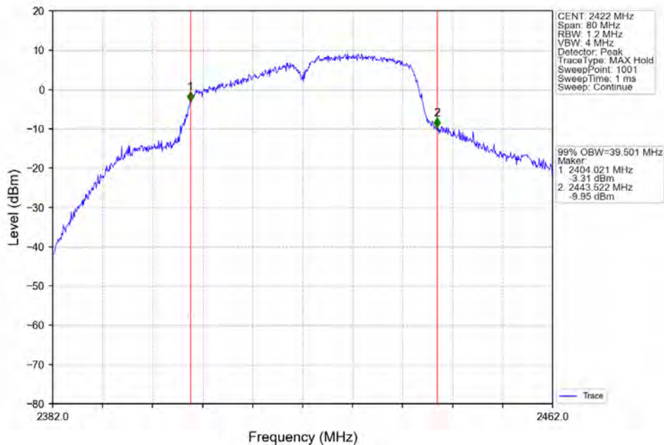
802.11n(HT40) LCH 2422MHz_Ant7 (SISO)_NTNV
