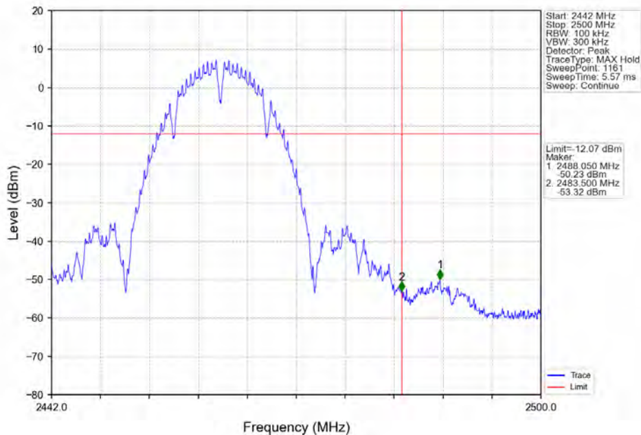
802.11b_HCH_2462MHz_Ant7 (SISO)_NTNV
