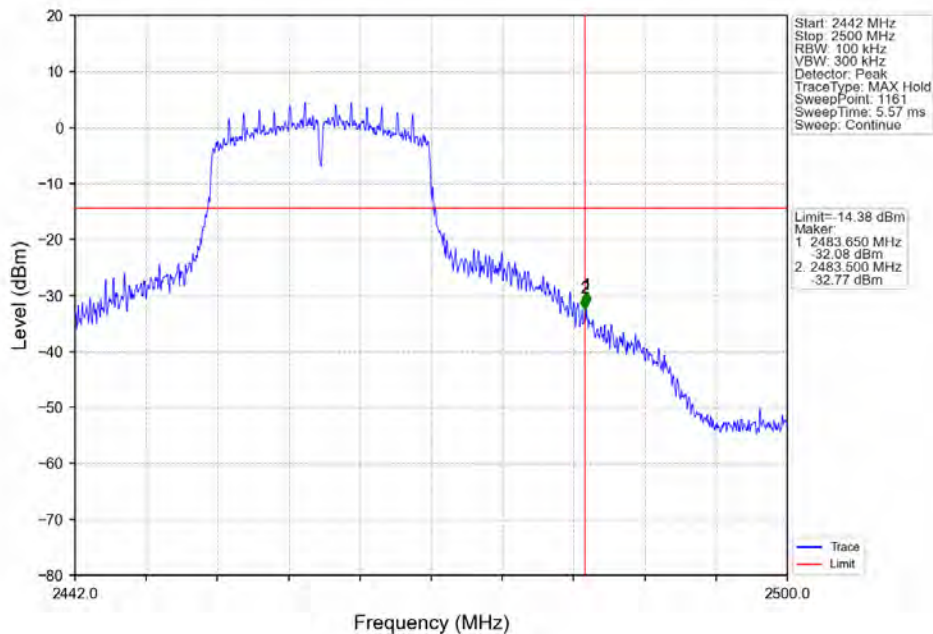
802.11n(HT20) HCH_2462MHz_Ant7 (SISO)_NTNV
