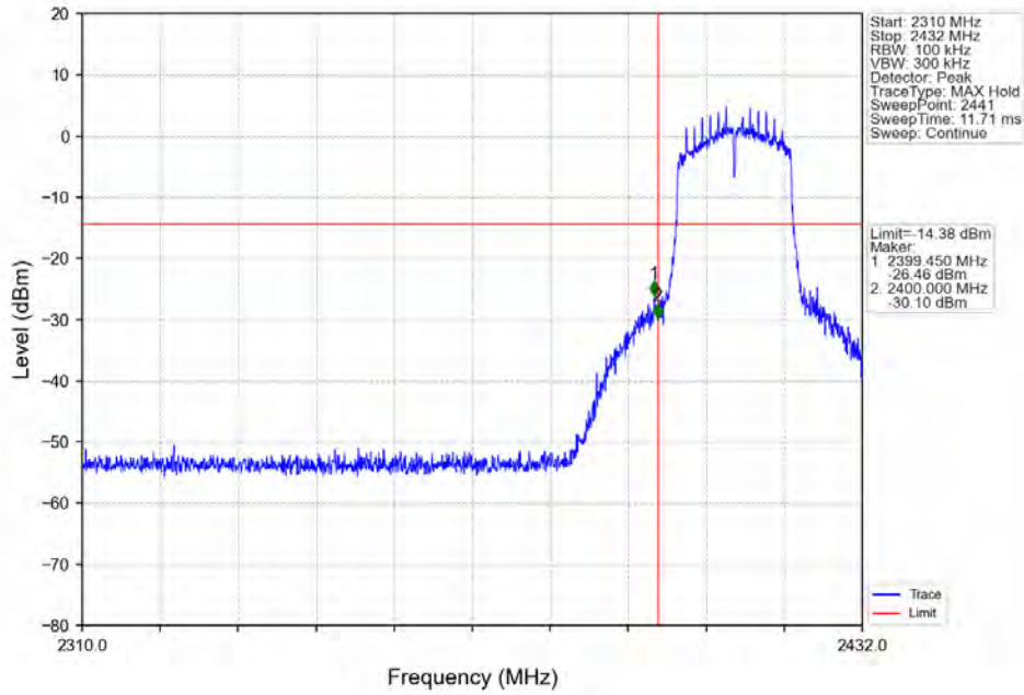
802.11n(HT20) LCH_2412MHz_Ant7 (SISO)_NTNV
