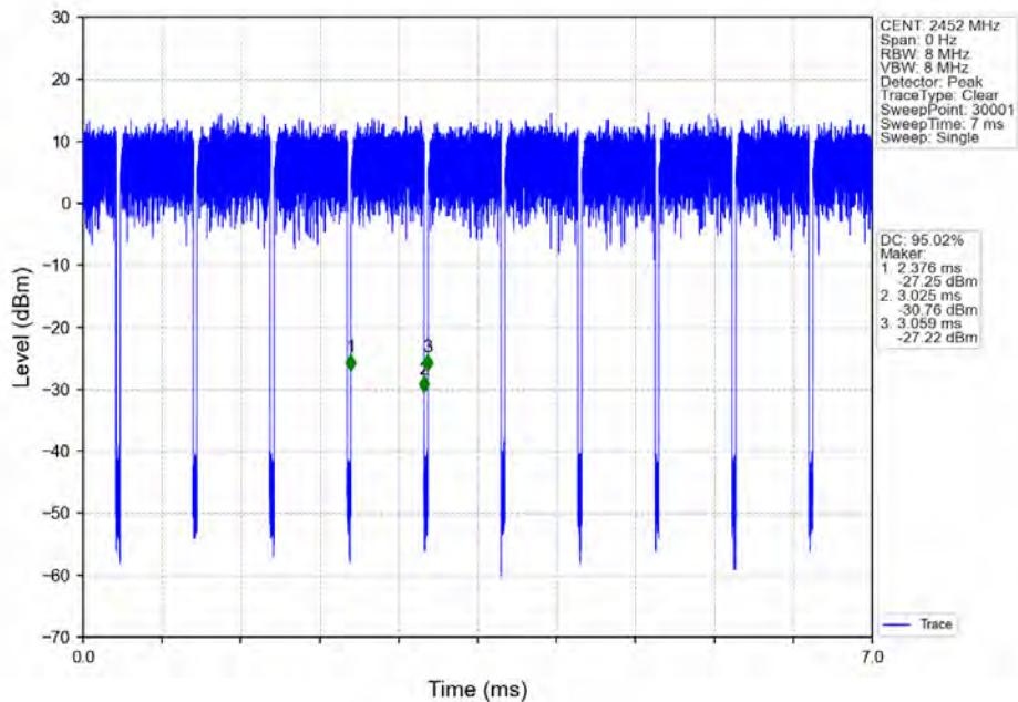
802.11n(HT40) HCH_2452MHz_Ant7 (SISO)_NTNV
