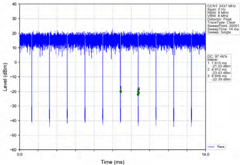
802.11n(HT20)_MCH_2437MHz_Ant7 (SISO)_NTNV
