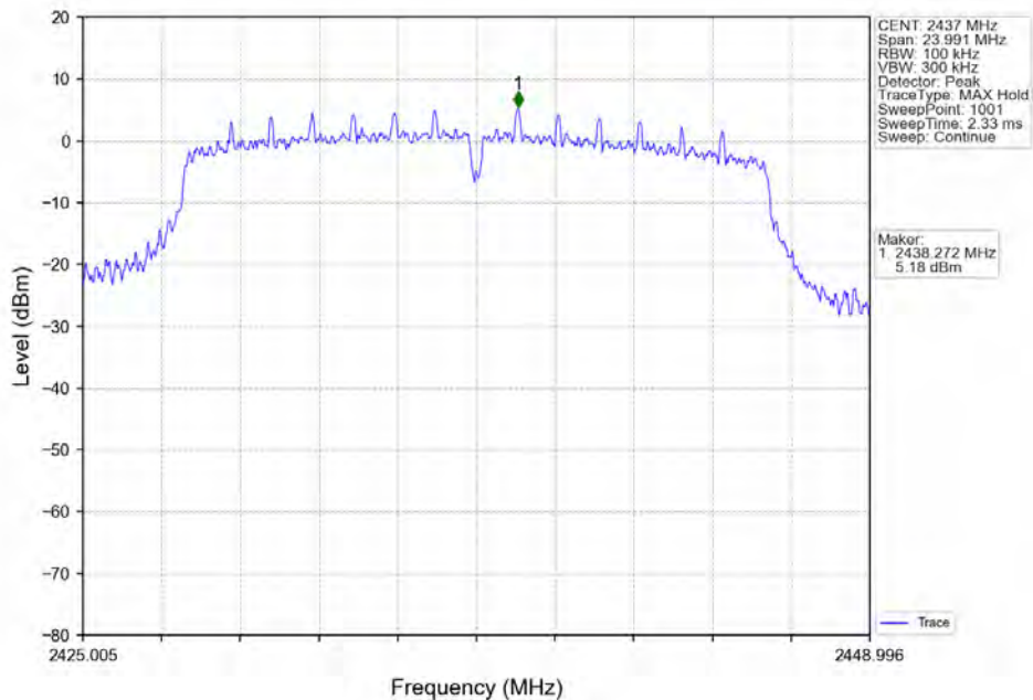
802.11n(HT20)_MCH_2437MHz_Ant7 (SISO)_NTNV
