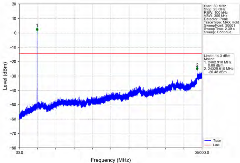
802.11g_HCH_2462MHz_Ant7 (SISO)_NTNV
