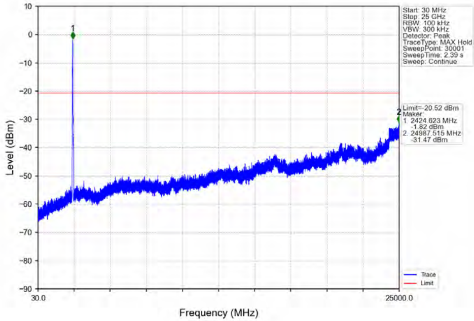
802.11n(HT40)_MCH_2437MHz_Ant7 (SISO)_NTNV
