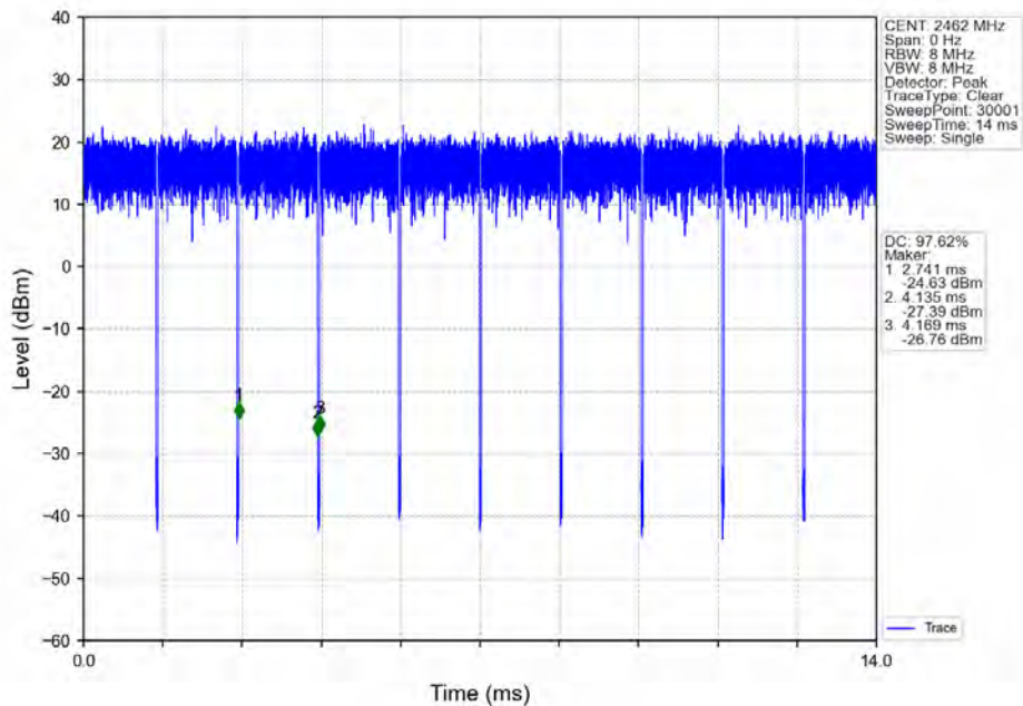
802.11g_HCH_2462MHz_Ant7 (SISO)_NTNV
