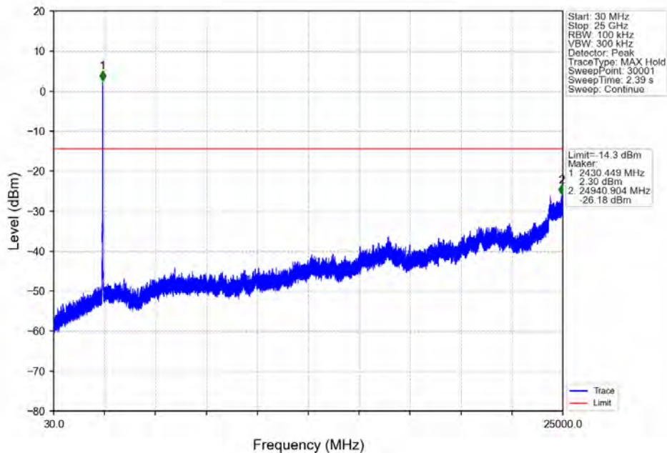
802.11g MCH 2437MHz Ant7 (SISO) NTVN
