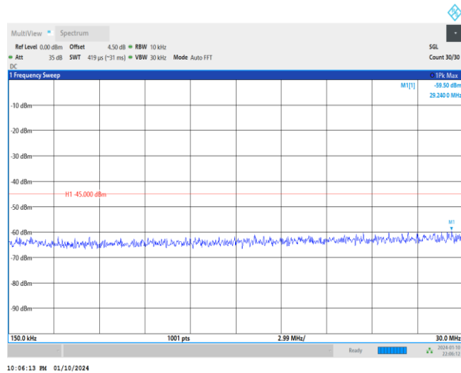
Band41-20MHz-QPSK-39750-1RB#0-Range2:0.15~30MHz
