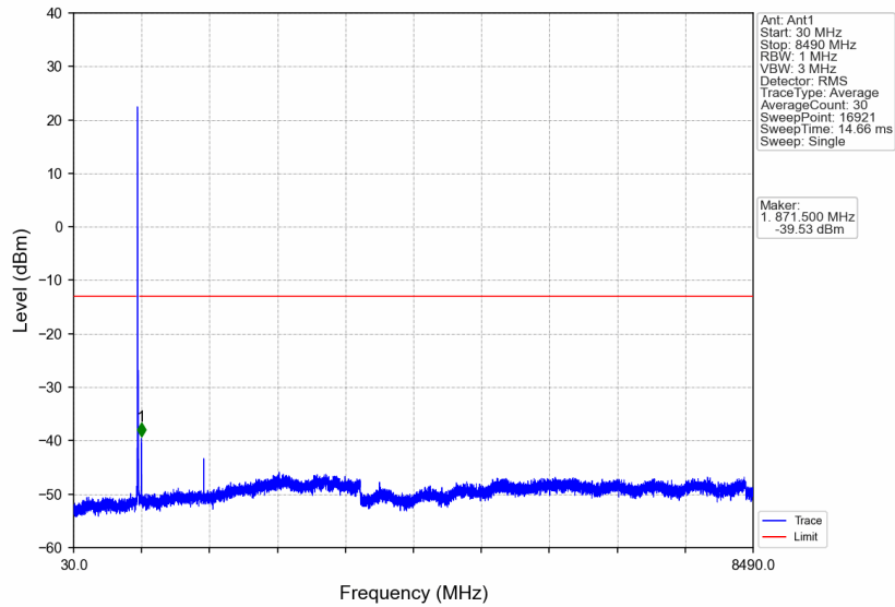
B26_10MHz_16QAM_LCH_829MHz_RB_50_0_NTNV
