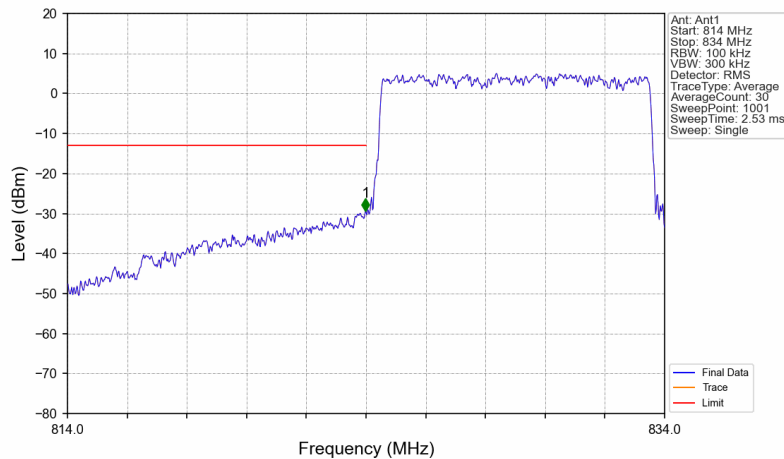
B26_10MHz_16QAM_LCH_829MHz_RB_50_0_NTNV
