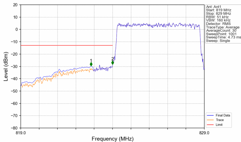
B26_5MHz_16QAM_LCH_826.5MHz_RB_25_0_NTNV
