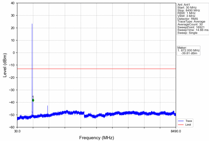
B26_5MHz_16QAM_LCH_826.5MHz_RB_25_0_NTNV
