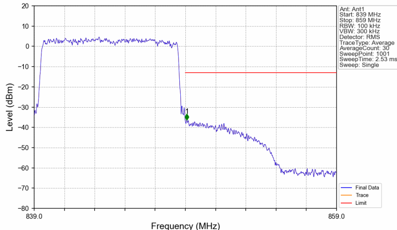
B26_10MHz_64QAM_HCH_844MHz_RB_50_0_NTNV
