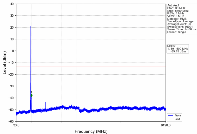
B26_10MHz_16QAM_HCH_844MHz_RB_1_0_NTNV
