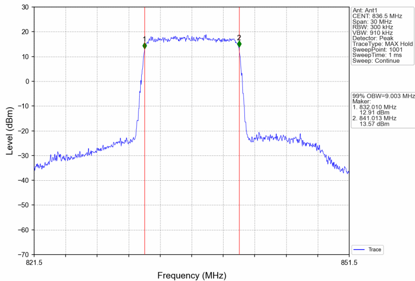
B26_10MHz_16QAM_MCH_836.5MHz_RB_50_0_NTNV
