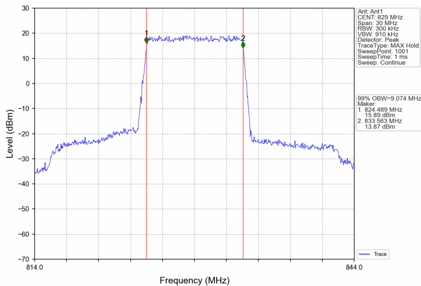
B26_10MHz_QPSK_LCH_829MHz_RB_50_0_NTNV
