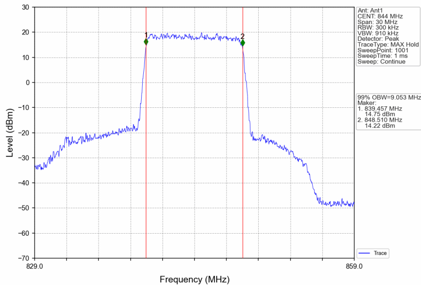
B26_10MHz_QPSK_HCH_844MHz_RB_50_0_NTNV
