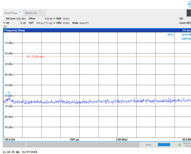
Band25-20MHz-QPSK-26140-1RB#0-Range2:0.15~30MHz
