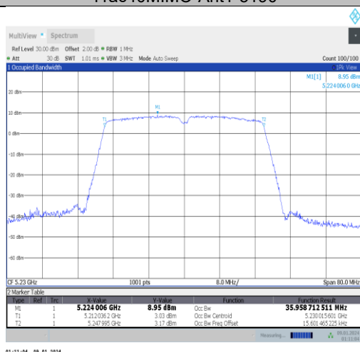
11ac40MIMO-Ant1-5230
