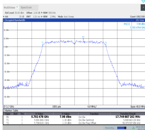
11ac20MIMO-Ant0-5700
