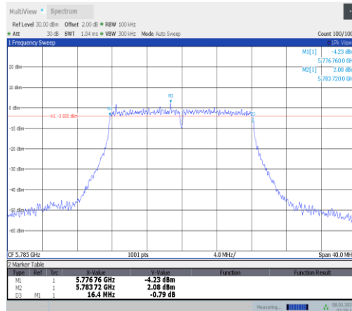
11a-Ant0-5785-PASS
