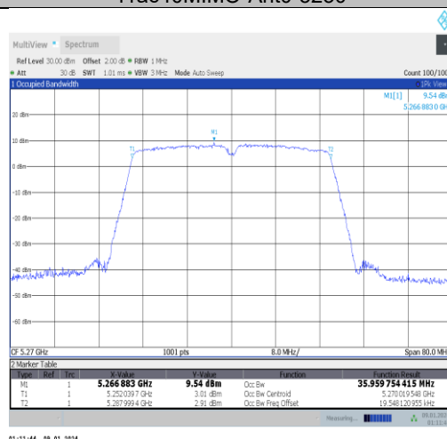
11ac40MIMO-Ant0-5270
