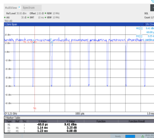
NTNV-11ac80MIMO-Ant1-5210
