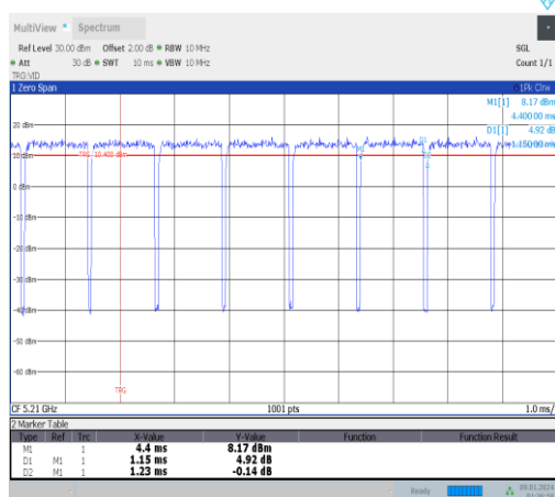
NTNV-11ac80MIMO-Ant0-5210
