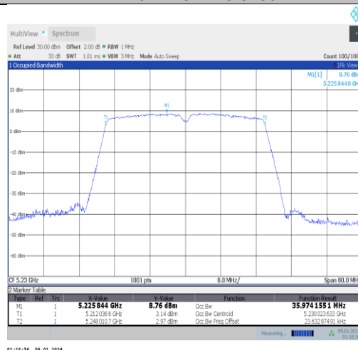
11ac40MIMO-Ant0-5230
