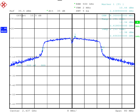
802.11n40_2437MHz 38.300MHz
