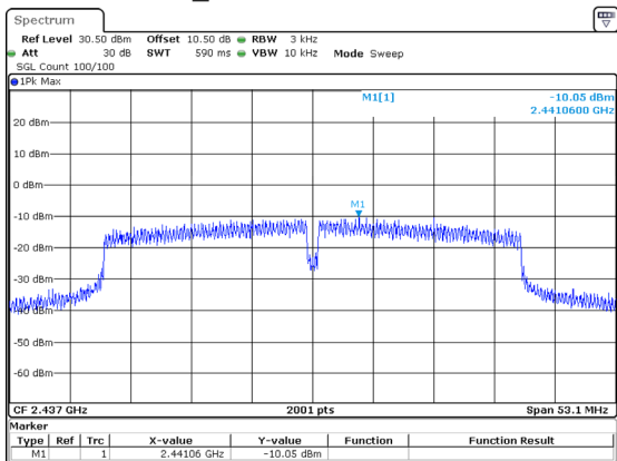
802.11n40_2437MHz -10.05dBm/3kHz
