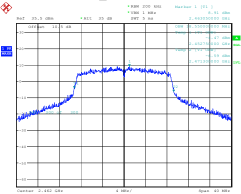
802.11n20_2462MHz 18.550MHz
