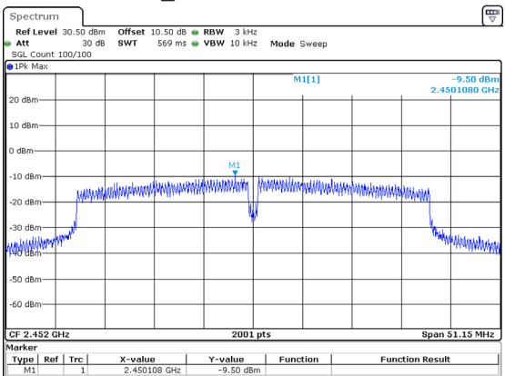
802.11n40_2452MHz -9.50dBm/3kHz
