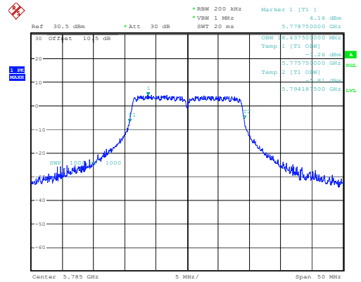
802.11ac20_5785MHz 18.438MHz
