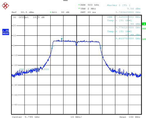
802.11ac40_5795MHz 37.625MHz
