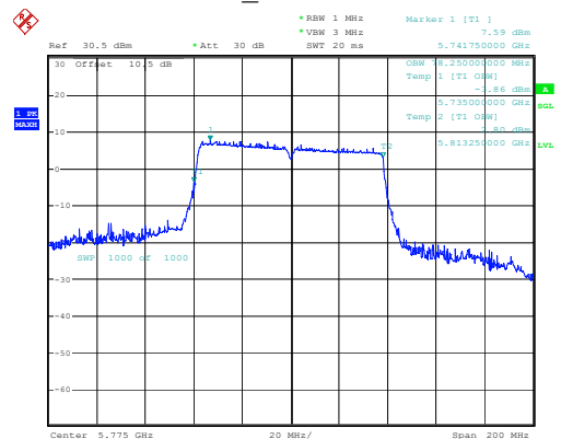
802.11ac80_5775MHz 78.250MHz
