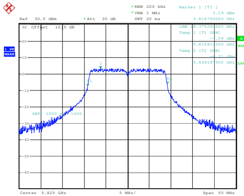
802.11ac20_5825MHz 18.375MHz
