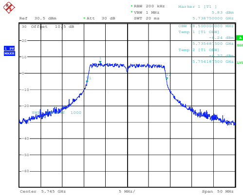
802.11ac20_5745MHz 18.500MHz
