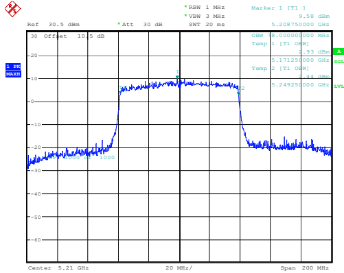
802.11ax80_5210MHz_RU_Full 78MHz
