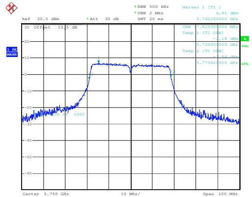
802.11ac40_5755MHz 37.625MHz
