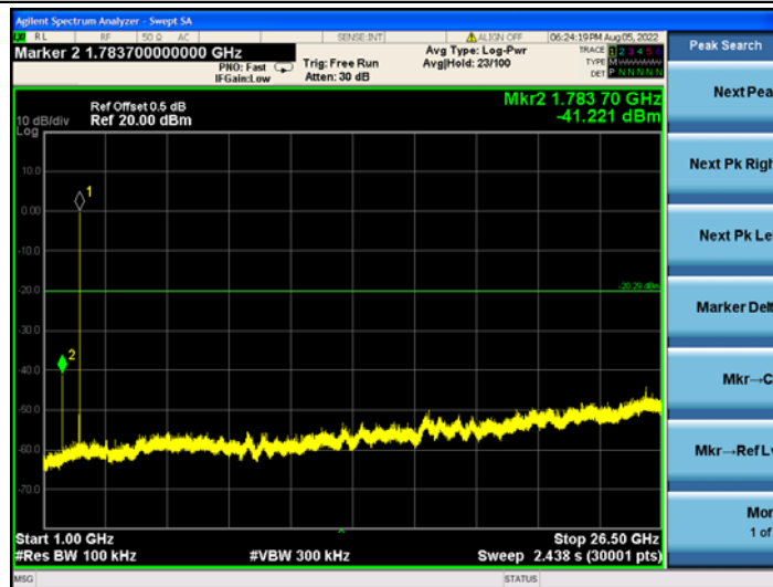
BLE_2480_1000~26500
