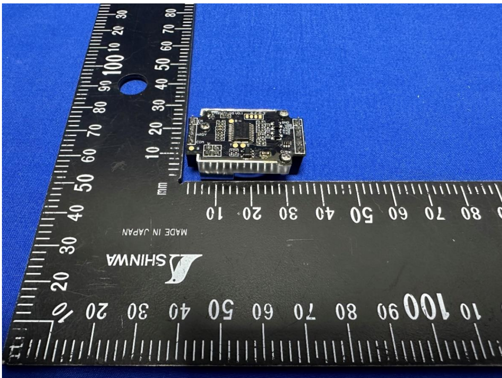
(8) EUT Photo
