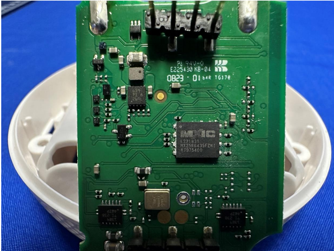
(11)EUT Photo
