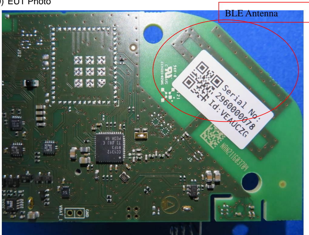
(10) EUT Photo
