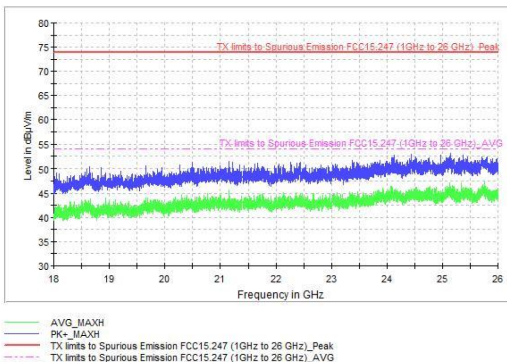
18GHz_26GHz_VP_CH High
