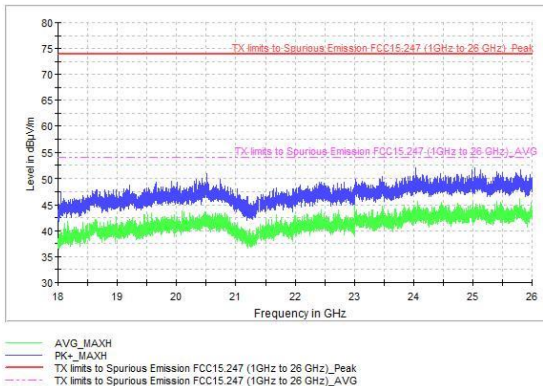
18GHz_26GHz_VP_CH Low
