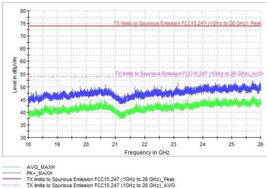
18GHz_26GHz_HP_CH Low
