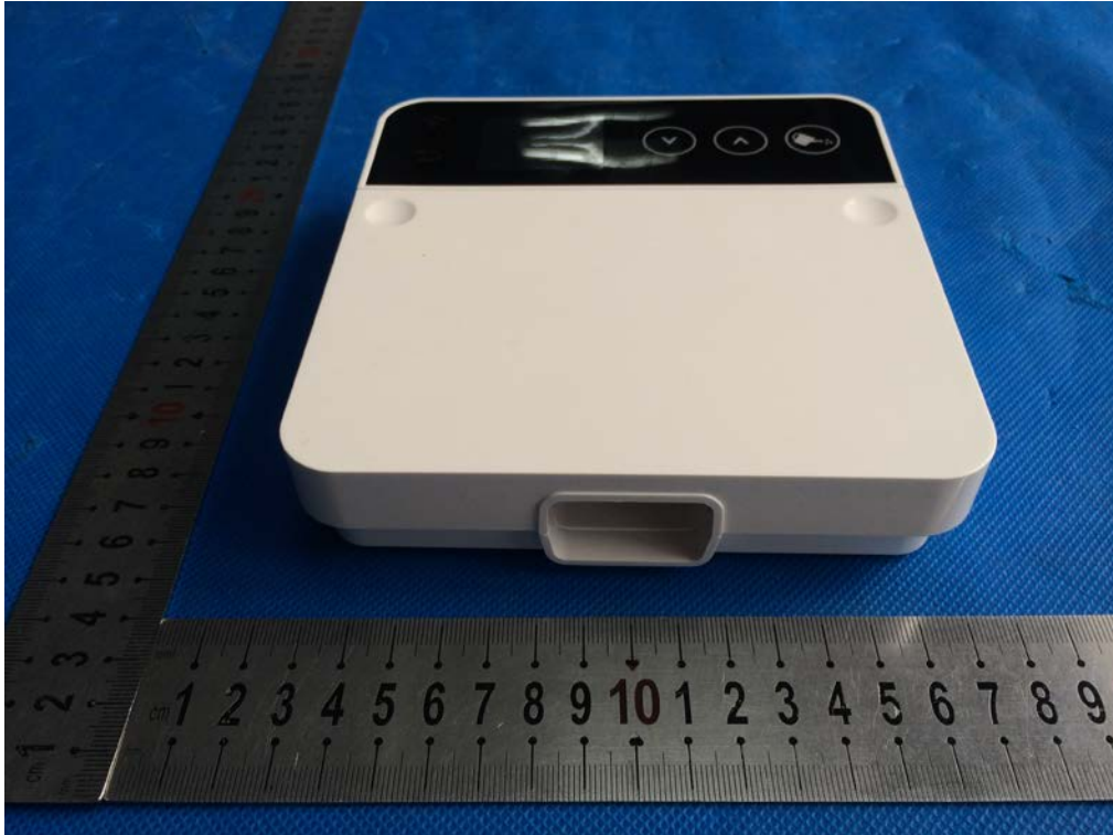
EUT –View 4
