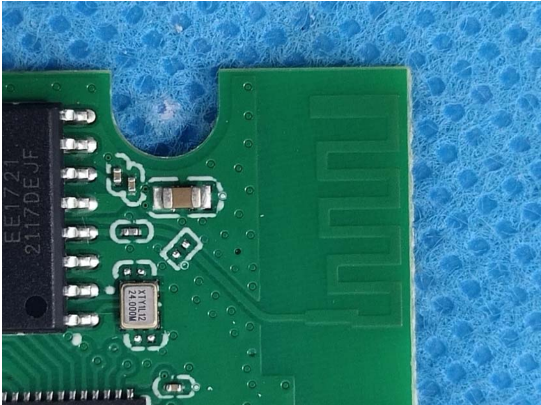
BLE Antenna
