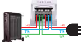
4.2 控制单火线开关正确接线方法 (比如灯具开关)。
