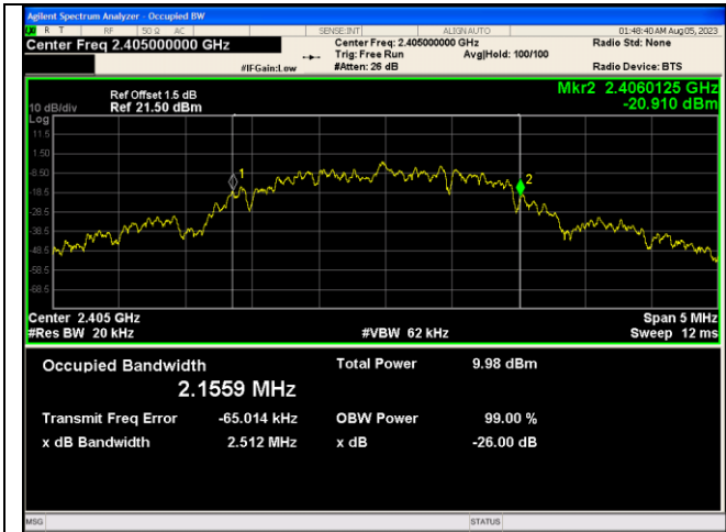
Zigbee 2405
