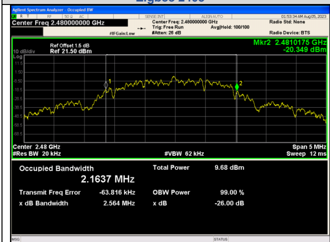
Zigbee 2480
