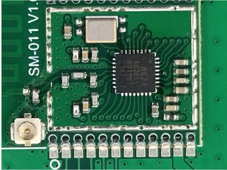
BLT/WiFi chip
