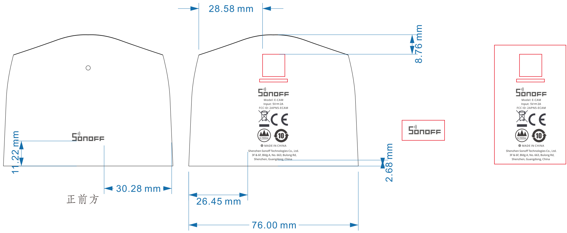
镭雕位置
