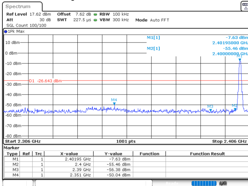
Band Edge NVNT BLE 2402MHz Ant1 Emission
