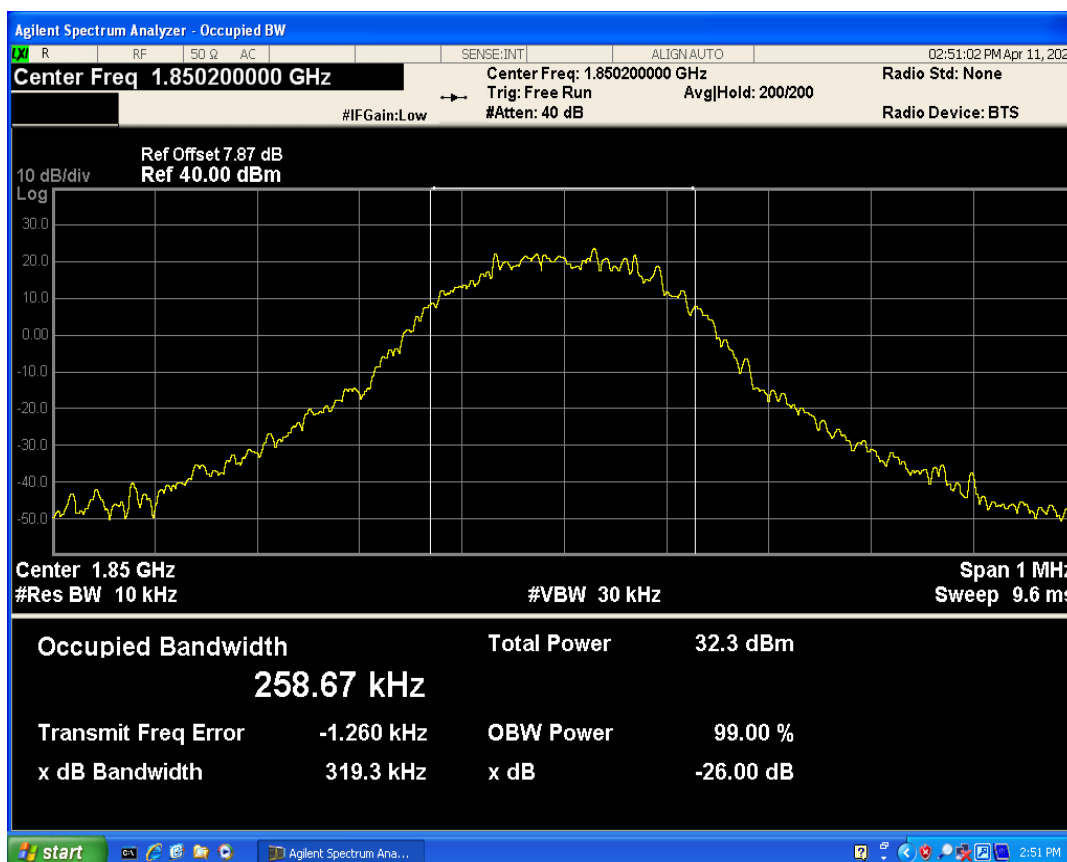
EGPRS1900 Channel=512
