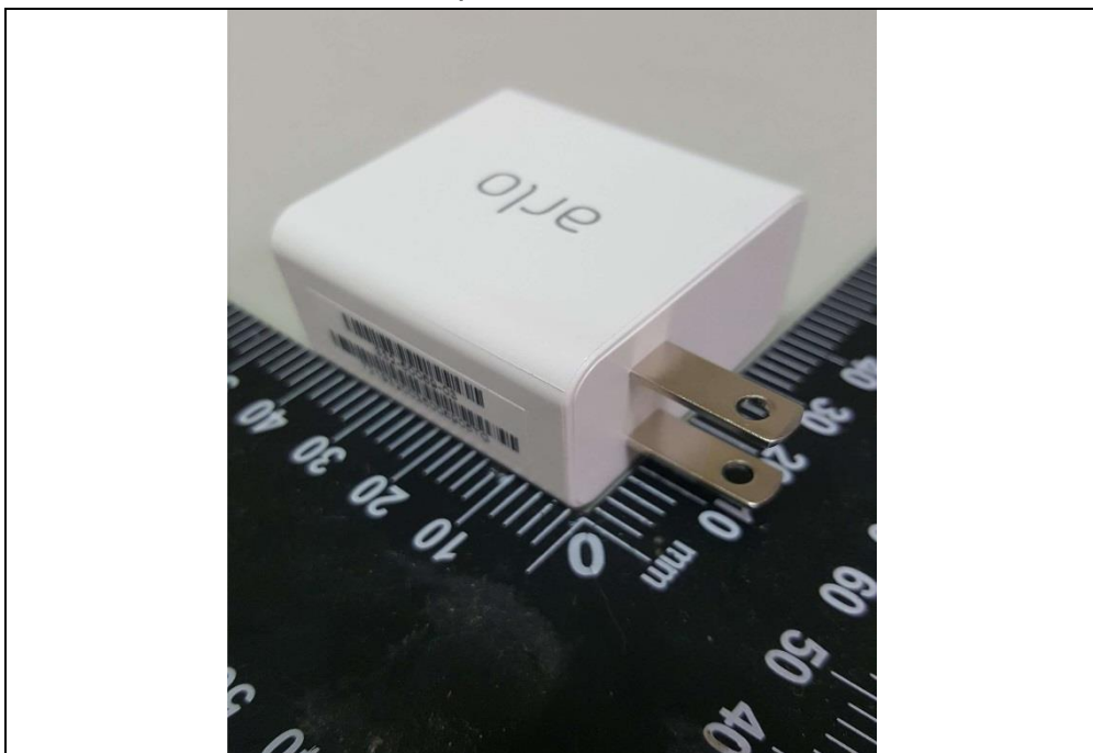
Adapter: 2ADB010B
