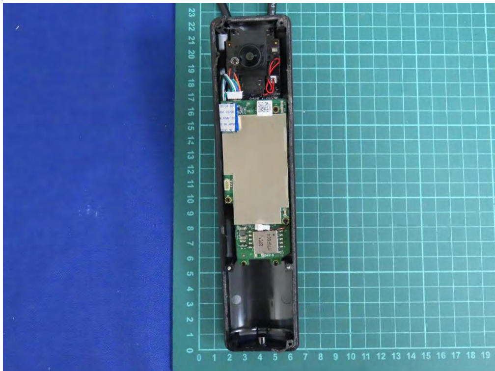
(48) EUT Photo
