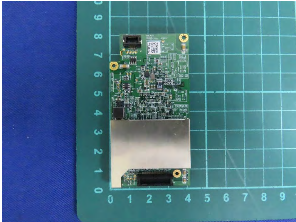
(59) EUT Photo
