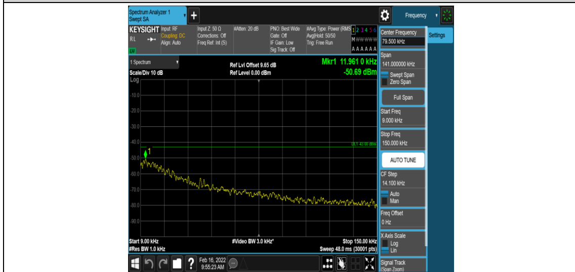
Band66-5MHz-QPSK-132322-1-0-Low-0.009-0.15--50.69-PASS
