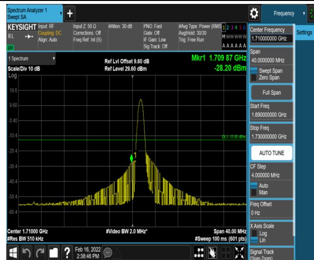
Band66-20MHz-16QAM-132072-1-0-Low--28.20-PASS
