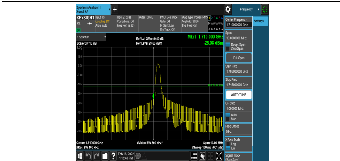
Band66-5MHz-16QAM-131997-1-0-Low--26.08-PASS
