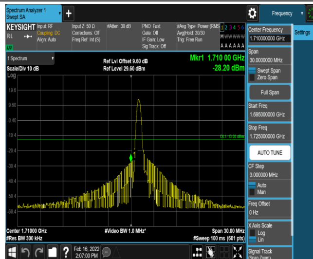
Band66-15MHz-16QAM-132047-1-0-Low--28.20-PASS
