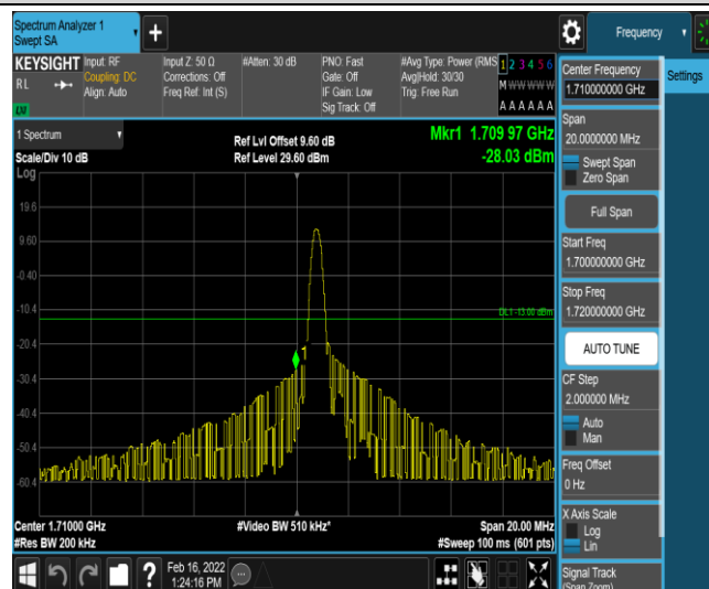
Band66-10MHz-16QAM-132022-1-0-Low--28.03-PASS
