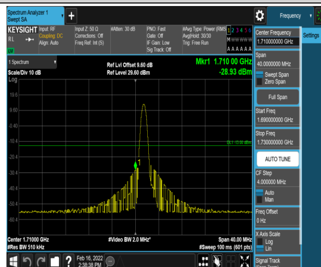
Band66-20MHz-QPSK-132072-1-0-Low--28.93-PASS
