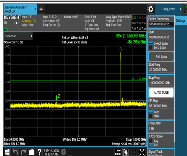
Band26-3MHz-16QAM-26740-1-0-Low-30-1000--35.2-PASS
