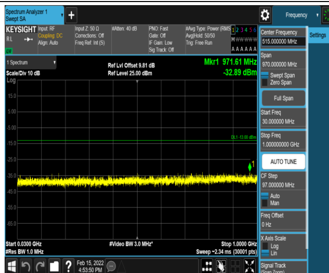
Band25-20MHz-QPSK-26365-1-0-Low-30-1000--32.89-PASS
