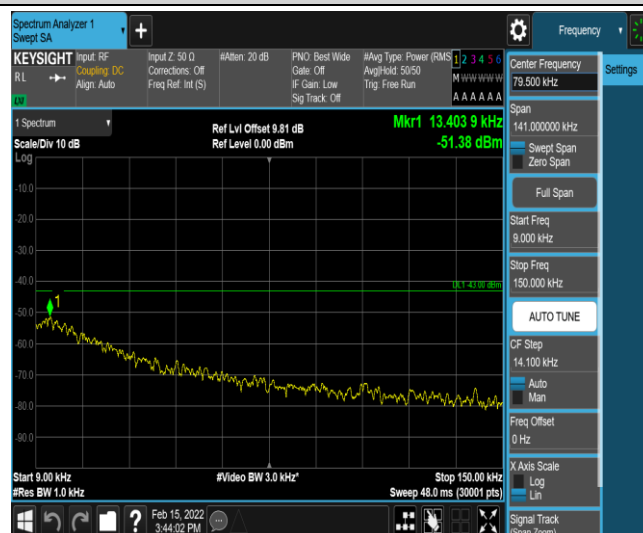
Band25-3MHz-QPSK-26365-1-0-Low-0.009-0.15--51.38-PASS
