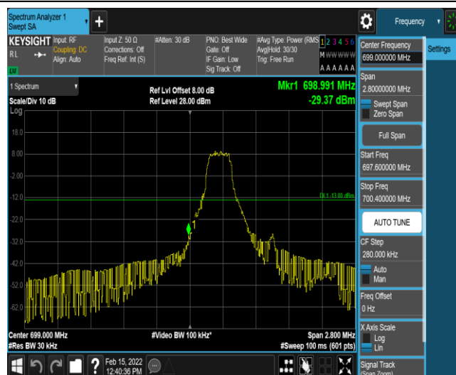
Band12-1.4MHz-16QAM-23017-1-0-Low--29.37-PASS
