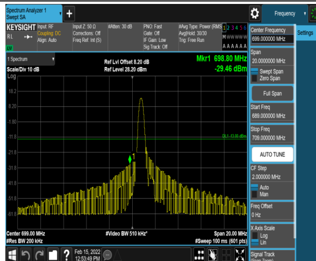
Band12-10MHz-16QAM-23060-1-0-Low--29.46-PASS
