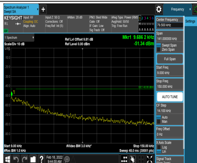
Band2-20MHz-QPSK-18700-1-0-Low-0.009-0.15--51.34-PASS
