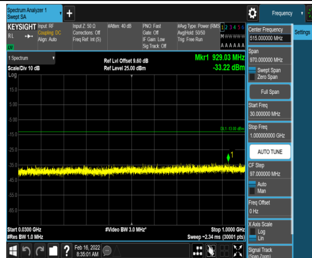
Band66-3MHz-QPSK-131987-1-0-Low-30-1000--33.22-PASS
