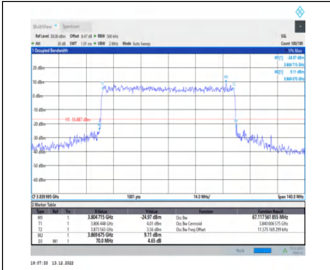
1-N77-3700-3980-30-70-M-7-CP-16QAM-Outer_Full-189@0-Ant1-67.118-70.000-≤70-PASS
