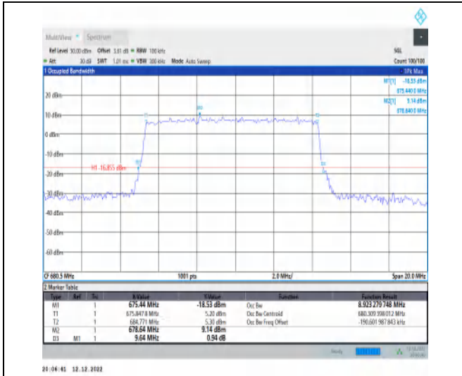
1-N71-15-10-M-5-DFT-256QAM-Outer_Full-50@0-A nt1-8.923-9.640-≤10-PASS
