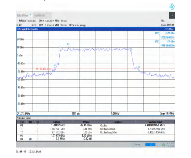
1-N66-15-5-L-6-CP-QPSK-Outer_Full-25@0-Ant1-4. 481-5.300-≤5-PASS
