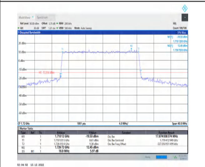
1-N66-15-20-L-3-DFT-16QAM-Outer_Full-100@0-Ant 1-17.875-18.800-≤20-PASS
