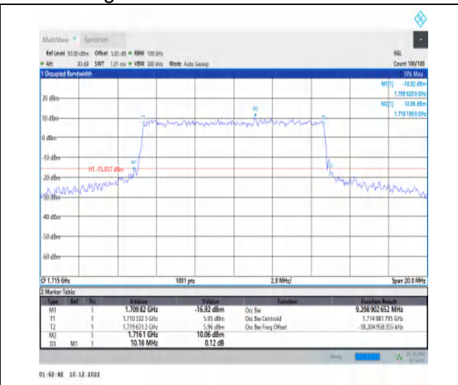
1-N66-15-10-L-7-CP-16QAM-Outer_Full-52@0-Ant1 -9.299-10.160-≤10-PASS
