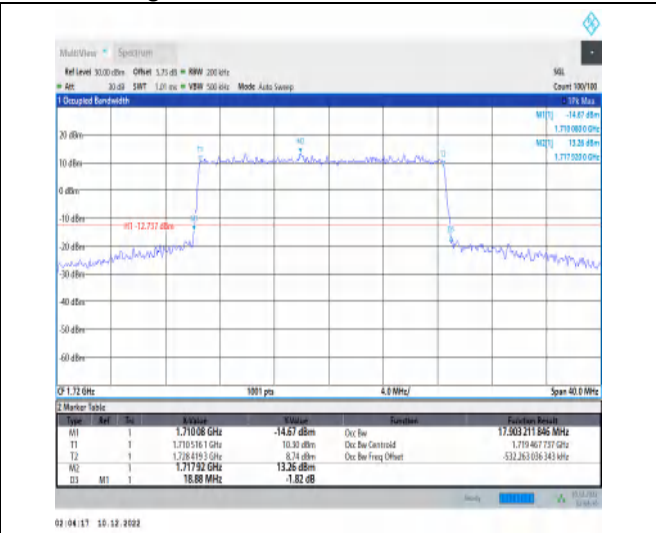
1-N66-15-20-L-1-DFT-QPSK-Outer_Full-100@0-Ant 1-17.903-18.880-≤20-PASS
