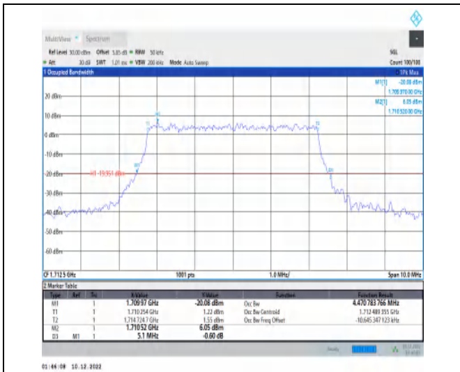
1-N66-15-5-L-9-CP-256QAM-Outer_Full-25@0-Ant1 -4.471-5.100-≤5-PASS
