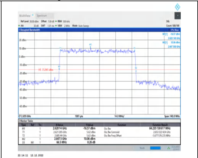
1-N41-30-70-H-5-DFT-256QAM-Outer_Full-180@0-A nt1-64.235-66.500- \leq 70 -PASS
