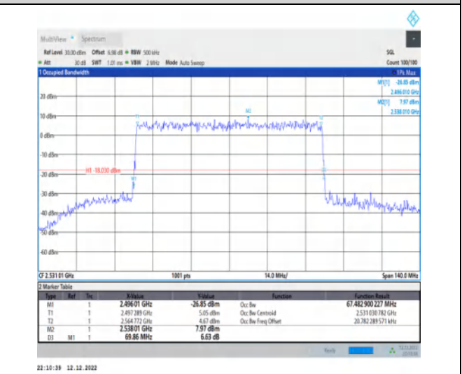
1-N41-30-70-L-9-CP-256QAM-Outer_Full-189@0-Ant1 t1-67.483-69.860-≤70-PASS
