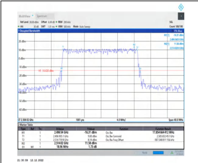
1-N41-30-20-L-5-DFT-256QAM-Outer_Full-50@0-A nt1-17.855-18.960-≤20-PASS
