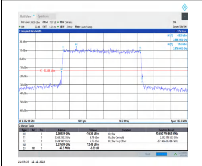
1-N41-30-50-M-5-DFT-256QAM-Outer_Full-128@0-A Ant1-45.651-47.500-≤50-PASS
