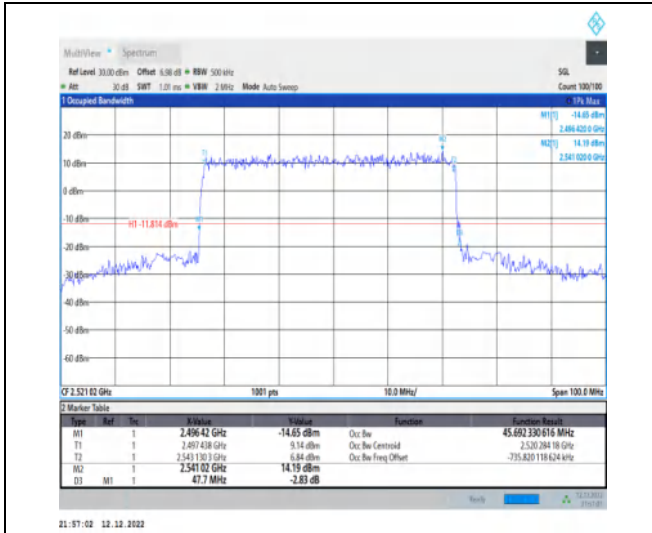
1-N41-30-50-L-4-DFT-64QAM-Outer_Full-128@0-A nt1-45.692-47.700-≤50-PASS
