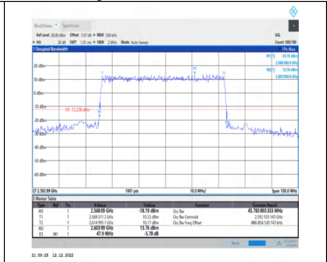
1-N41-30-50-M-4-DFT-64QAM-Outer_Full-128@0-A nt1-45.784-47.900-≤50-PASS
