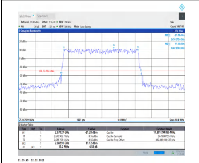
1-N41-30-20-H-5-DFT-256QAM-Outer_Full-50@0-A nt1-17.802-19.200-≤20-PASS
