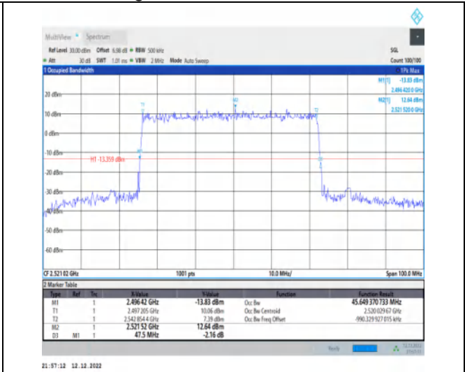
1-N41-30-50-L-5-DFT-256QAM-Outer_Full-128@0-A nt1-45.649-47.500-≤50-PASS
