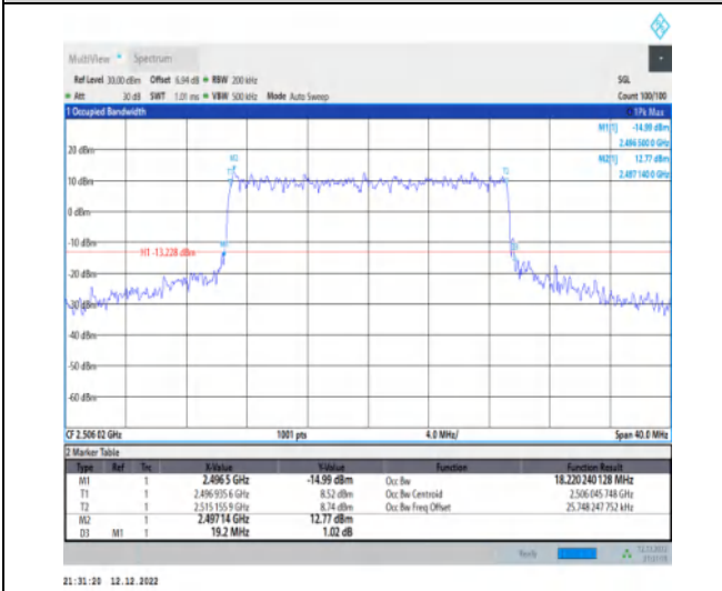
1-N41-30-20-L-7-CP-16QAM-Outer_Full-51@0-Ant1 -18.22-19.200-≤20-PASS
