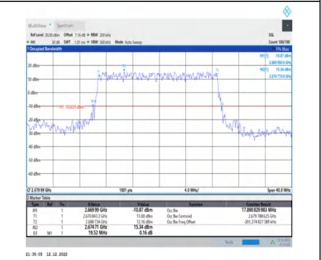
1-N41-30-20-H-2-DFT-PI2BPSK-Outer_Full-50@0-Ant1 -17.891-19.520-≤20-PASS
