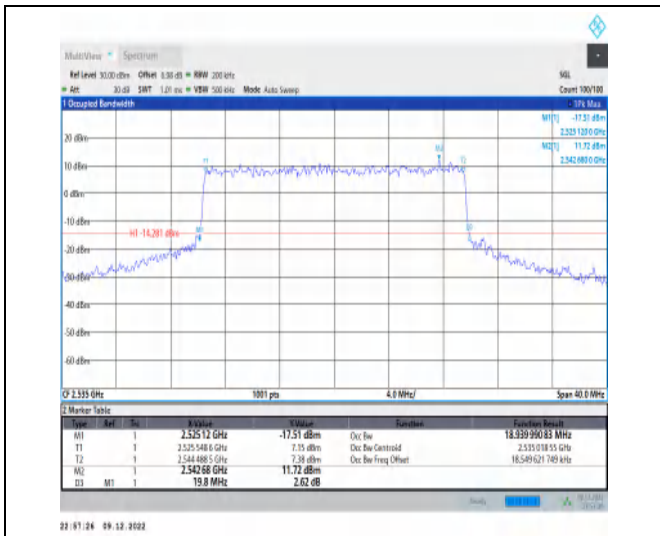
1-N7-15-20-M-7-CP-16QAM-Outer_Full-106@0-Ant1 -18.94-19.800-≤20-PASS
