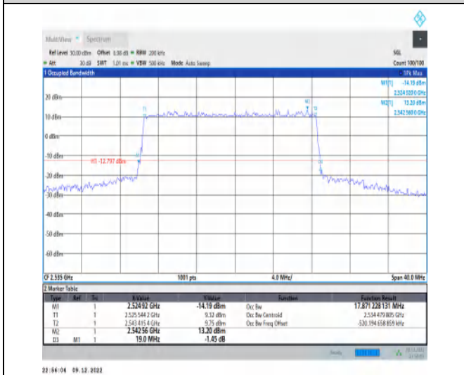
1-N7-15-20-M-1-DFT-QPSK-Outer_Full-100@0-Ant1 -17.871-19.000-≤20-PASS
