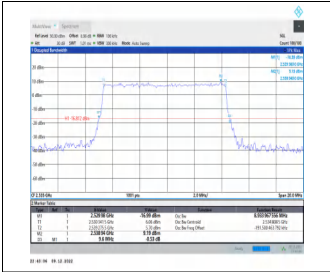
1-N7-15-10-M-5-DFT-256QAM-Outer_Full-50@0-Ant 1-8.934-9.600-≤10-PASS
