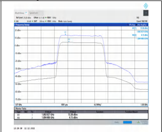
1-N2-PC3-15-20-H-2-CP-256QAM-Outer_Full-106@ 0-Ant1-9.23-100%-0.00-9.23-PASS-≤13
